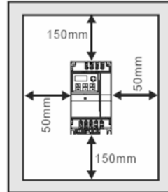
Метод установки В
