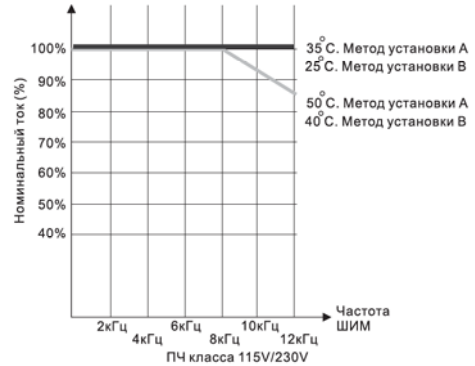
Метод установки А
