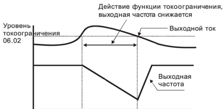
Токоограничение в установившемся режиме
