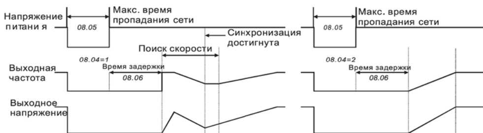
Рестарт после пропадания напряжения питания
