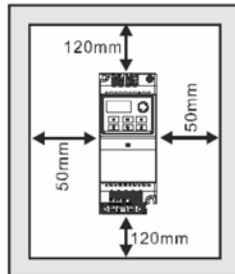
Метод установки В
