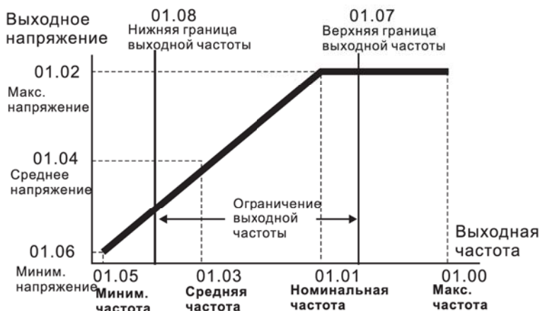
Типовая зависимость V/f
