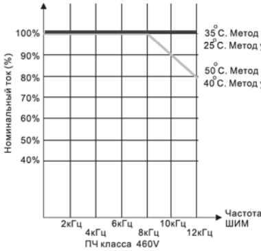
Типоразмер А
