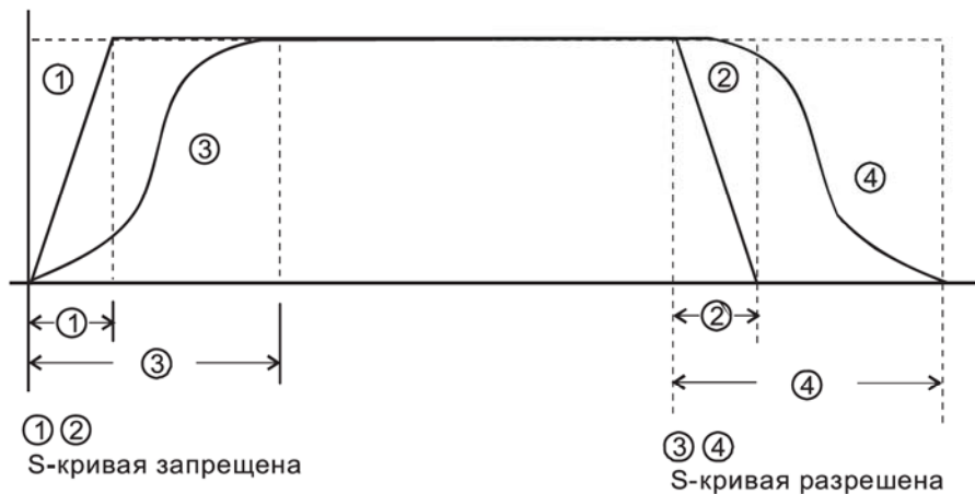
Характеристики разгона/торможения
