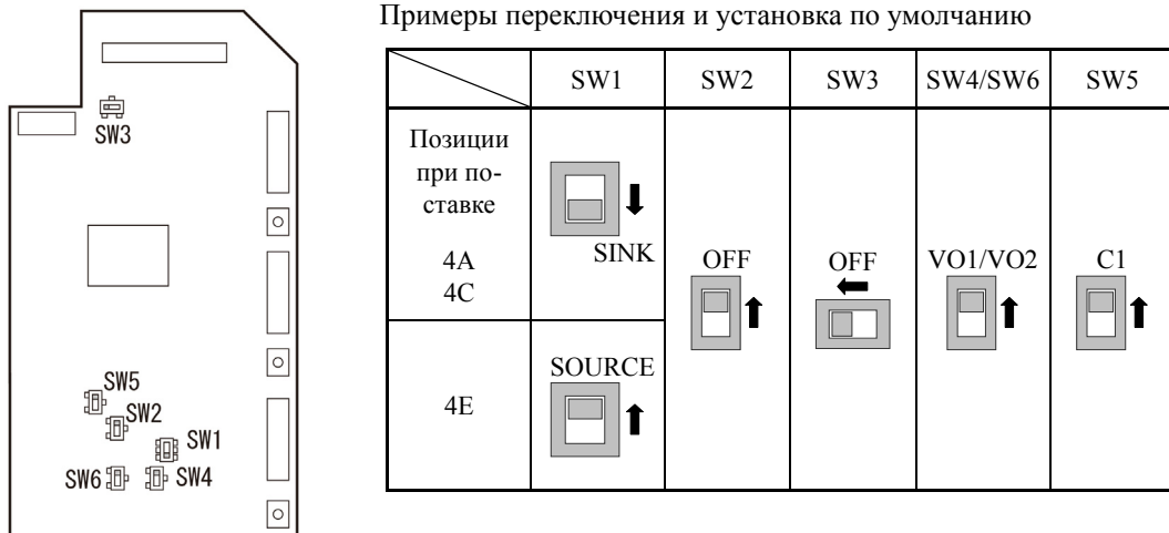
Рисунок 2.11 Расположение переключателей на печатной плате
