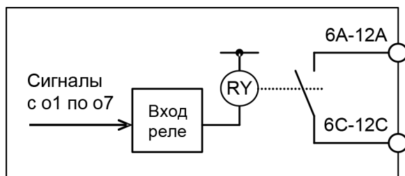
Рисунок 4.12 Внутренние цепи
